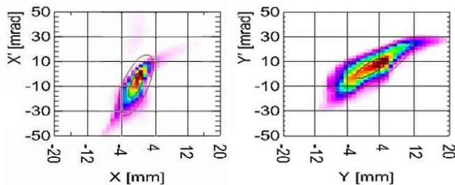
Figure 11: Émittances horizontale et verticale du faisceau d'1 mA d' O^{6+} obtenu avec PHOENIX 28 GHz V1.
