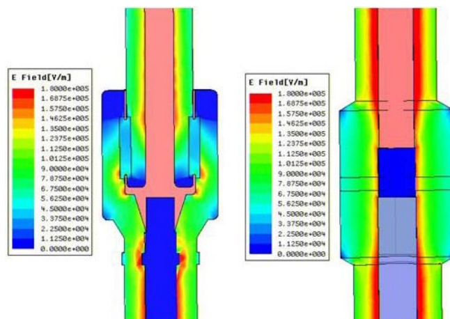
Figure 1 : Champ électrique pour une céramique cylindrique (à gauche) et pour une céramique disque (à droite) pour une puissance incidente 20 kW.
