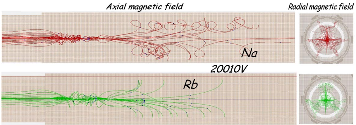
Figure 17: Calcul des trajectoires des ions 1+ sodium et rubidium prenant en compte les champs électriques et magnétiques.
