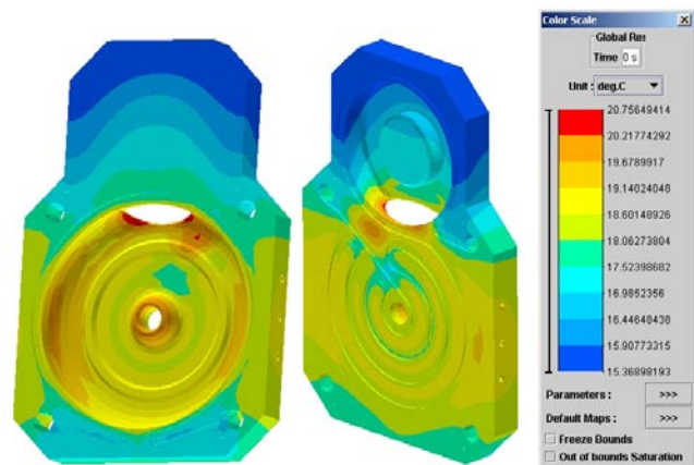
Figure 5: Cavités à couplage latéral. Étude thermique avec refroidissement. À gauche, on voit une cavité accélératrice, à droite une cavité de couplage, communicant par une fente de couplage.
