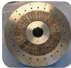
Figure 13: Tranche de structure hexapolaire 1,35 T et fin d'assemblage.
