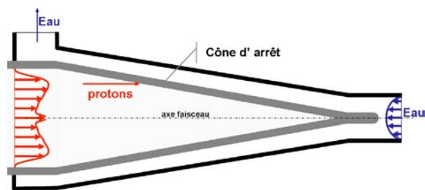
Figure 6 : Bloc d'arrêt faisceau de l'expérience IPHI.
