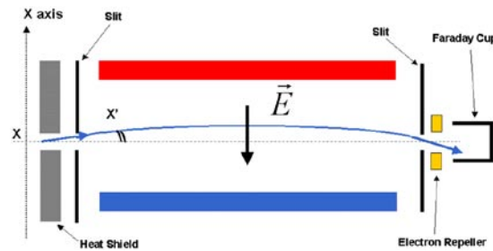
Figure 10: Schéma de principe des émittancemètres.
