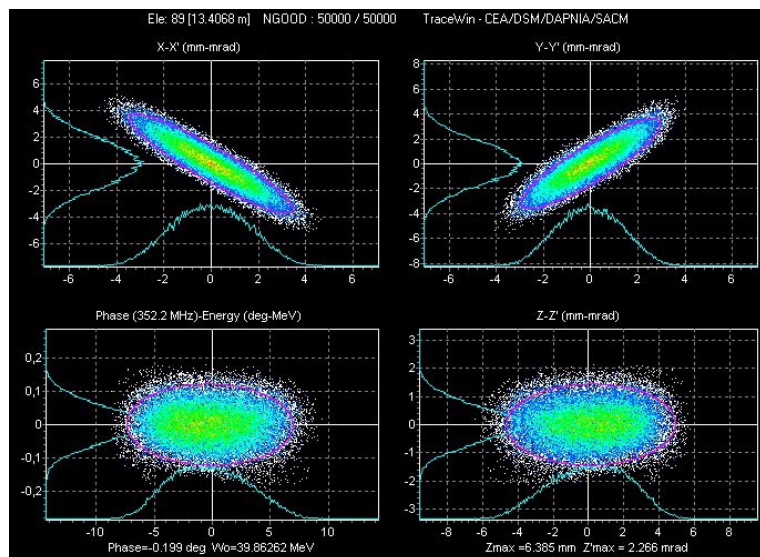
Figure 3: Émittance (longitudinale, transverse) d'un faisceau pulsé de protons de 65 mA en sortie du DTL.
