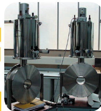
Figure 15: Bobines montées dans leurs cryostats.
