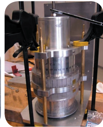
Figure 13: Tranche de structure hexapolaire 1,35 T et fin d'assemblage.
