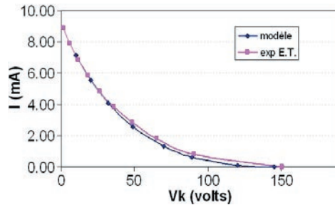
Figure 8 : Courbe de courant-tension caractéristique d'un canon à électrons. Comparaison expérience versus modèle théorique.
