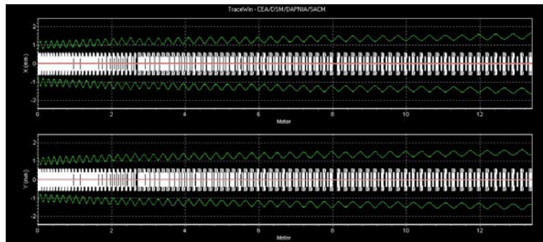
Figure 2: Enveloppe dans la direction x (haut) et y (bas) d'un faisceau pulsé de protons de 65 mA accéléré par le DTL en fonction de la position longitudinale dans le DTL.
