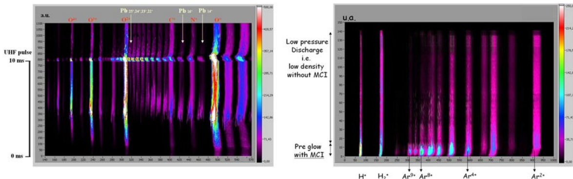
Figure 18: Spectres d'ions en mode afterglow-Pb et preglow-Ar (abscisse : champ B spectromètre, ordonnée : temps, couleur : intensité).
