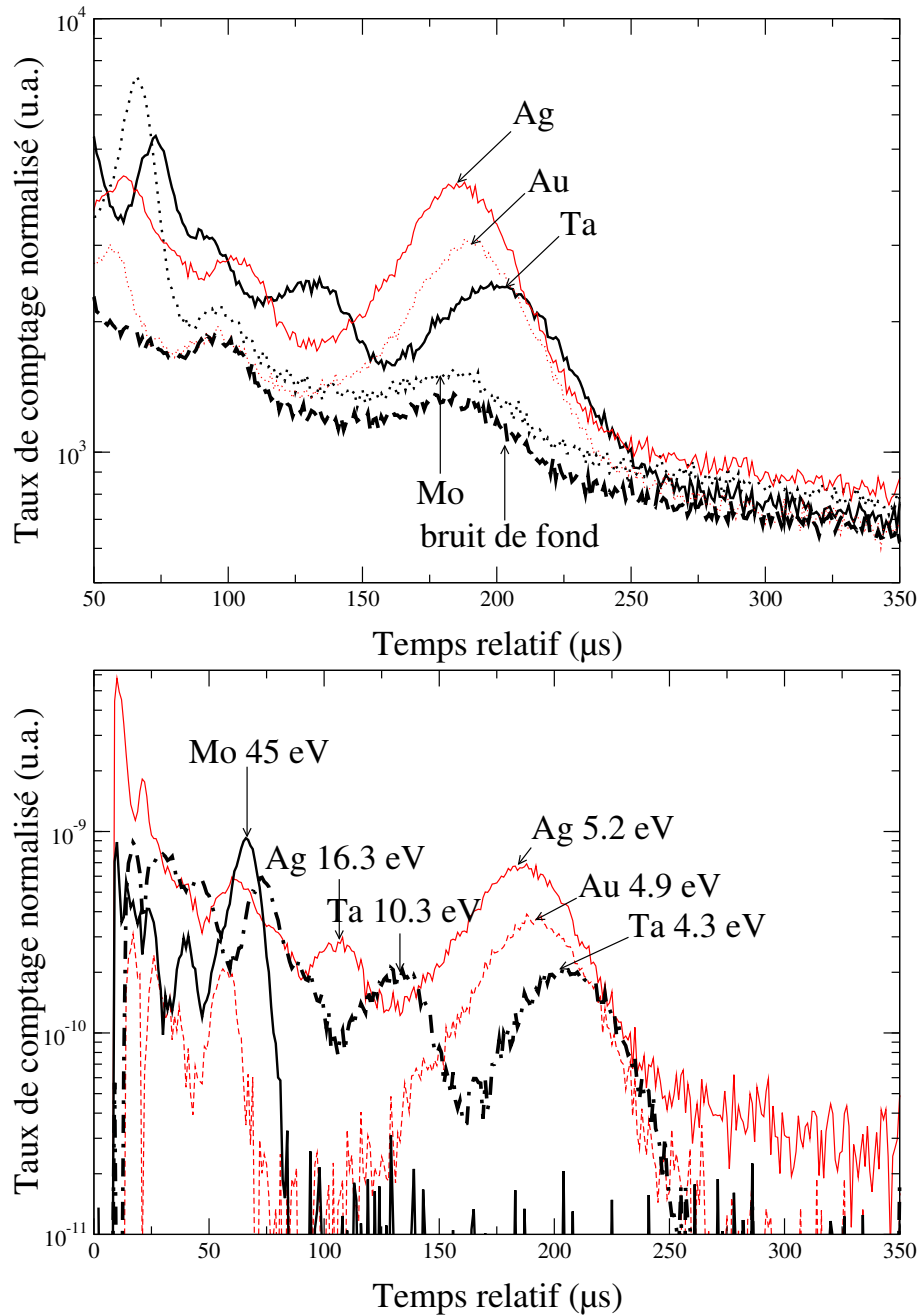
FIG. 8.9 – Spectres en temps relatif dans les scintillateurs YAP en double coïncidence, obtenus avec les cibles résonantes, normalisés au nombre de neutrons émis (en haut). Les spectres représentés dans la figure du bas correspondent aux spectres précédents après soustraction du bruit de fond.
