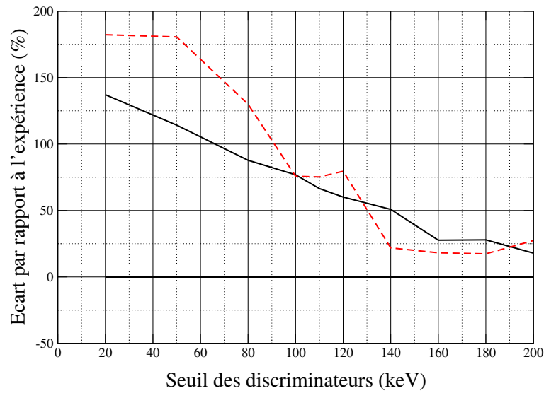
FIG. 8.12 – Ecart relatif des rapports \frac{\epsilon_{coinc\ double}}{\epsilon_{single}} (courbe pleine) et \frac{\epsilon_{coinc\ triple}}{\epsilon_{coincidence\ double}} (courbe pointillées), par rapport à ceux calculés expérimentalement. Les valeurs obtenues sont représentées pour le cas “2 mm”.
