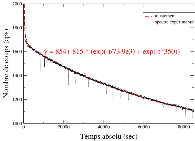
FIG. 7.2 – Exemple de décroissance du taux de comptage juste après une coupure du faisceau GENEPI.
