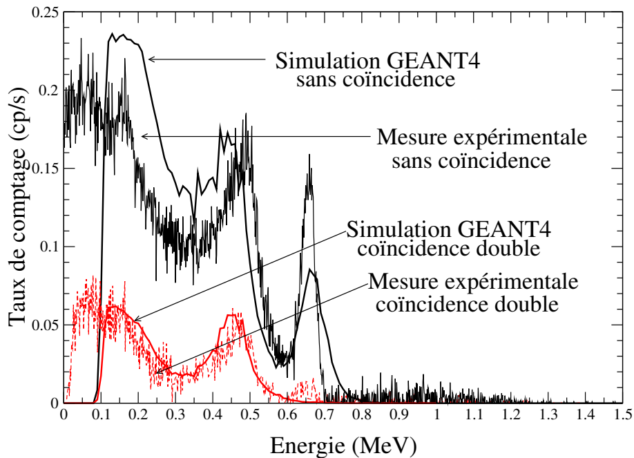
FIG. 6.7 – Comparaison entre le spectre en énergie d'un scintillateur YAP de 10 mm d'épaisseur avec une source de ^{137}\text{Cs} obtenu avec GEANT4 (courbe pleine), et le spectre expérimental (courbe pointillée), en fonction de la coïncidence.
