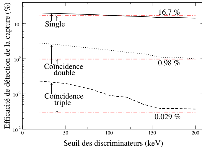
FIG. 8.11 – Efficacités de détection de la capture dans les scintillateurs YAP de 2 mm d’épaisseur en fonction de la coïncidence imposée, obtenues grâce à GEANT4. Les courbes constantes dont la valeur est spécifiée sur les graphiques correspond aux valeurs expérimentales.
