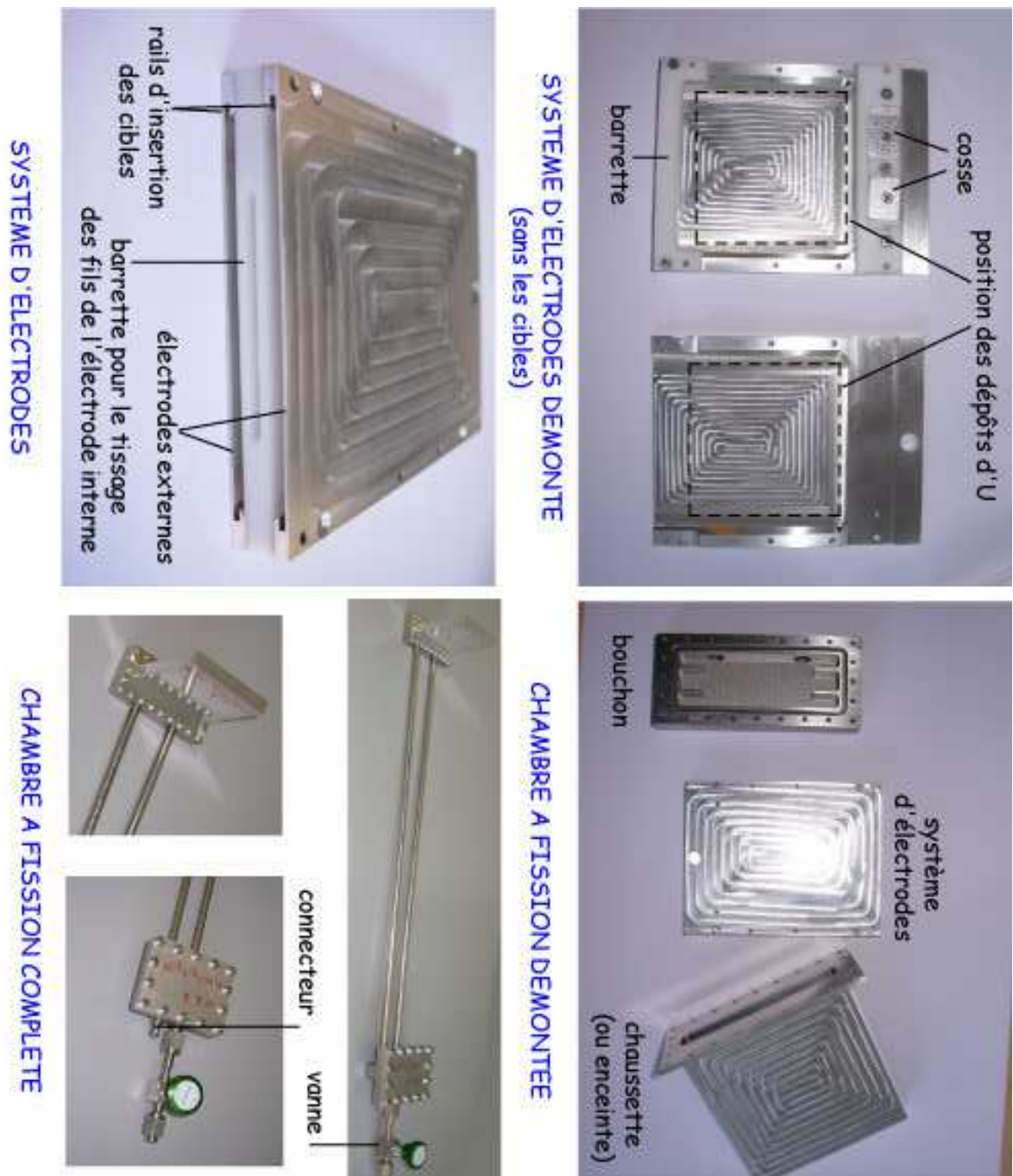
FIG. 4.12 – Photos de la chambre à fission démontée.
