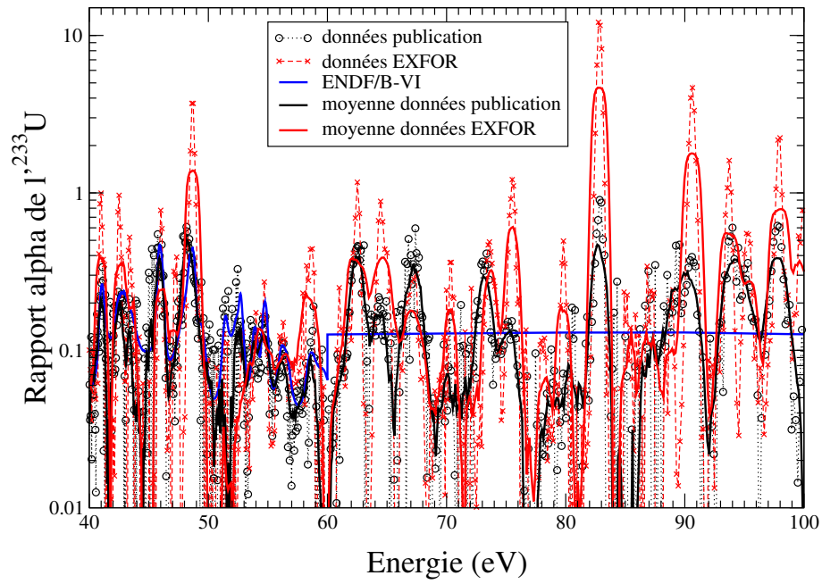
FIG. B.19 – Rapport \alpha de ^{233}\text{U} entre 40 eV et 100 eV.
