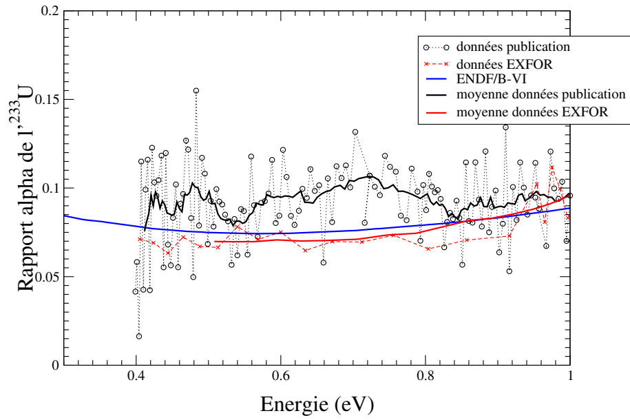
FIG. B.15 – Rapport \alpha de 1^{233}\text{U} entre 0.3 eV et 1 eV.
