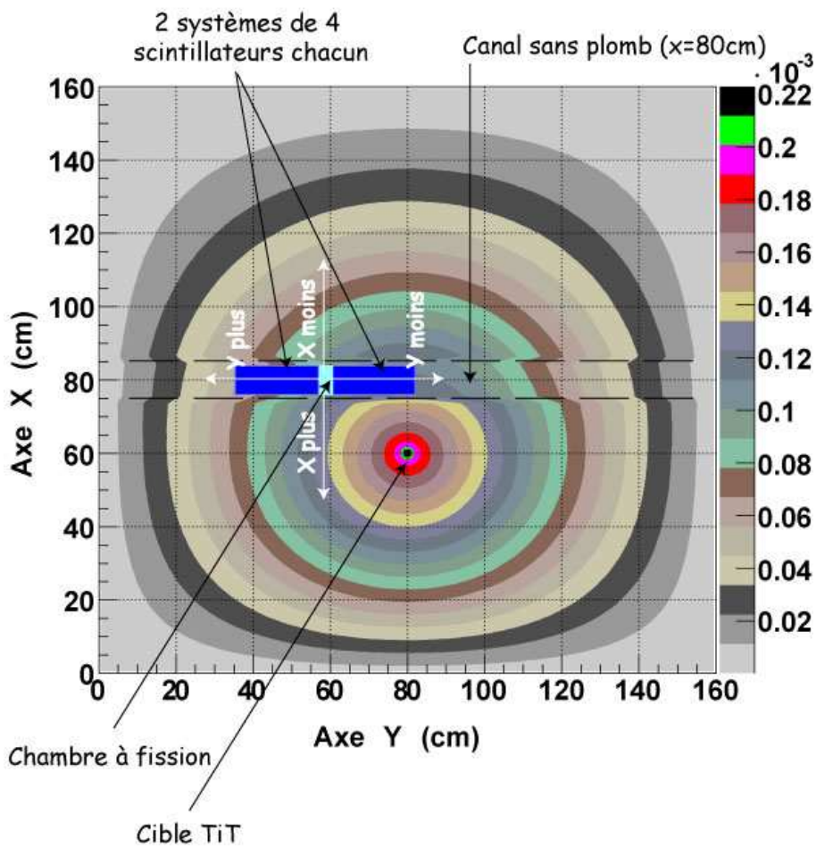
FIG. 9.7 – Taux de capture dans le bloc de plomb en fonction de la position X et Y, et intégré selon l'axe Z. Représentations en 3 dimensions (en haut) et en 2 dimensions (en bas).
