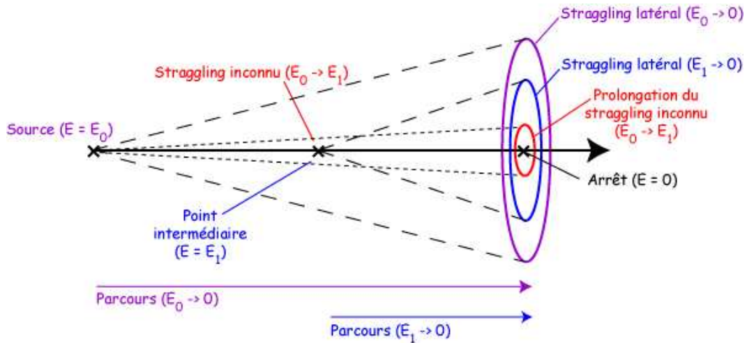
FIG. 5.10 – Représentation d’une trajectoire d’une particule et du stragglings latéral associé. La trajectoire de la particule est évaluée en trois points : à la source (énergie E_0 ), en un point intermédiaire (énergie E_1 ) et à la fin de son parcours (énergie nulle). Les stragglings latéraux sont également mentionnés.
