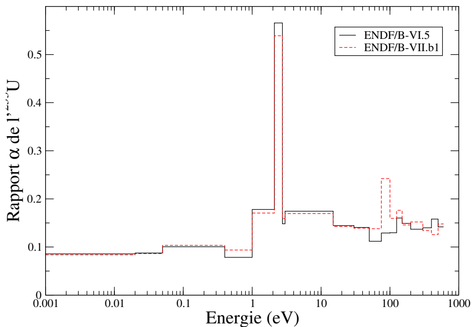
FIG. 2.9 – Comparaison entre la bibliothèque ENDF/B-VI.5 (2001) et sa nouvelle version ENDF/B-VII.b1 (2006), pour le rapport \alpha de l' ^{233}\text{U} .
