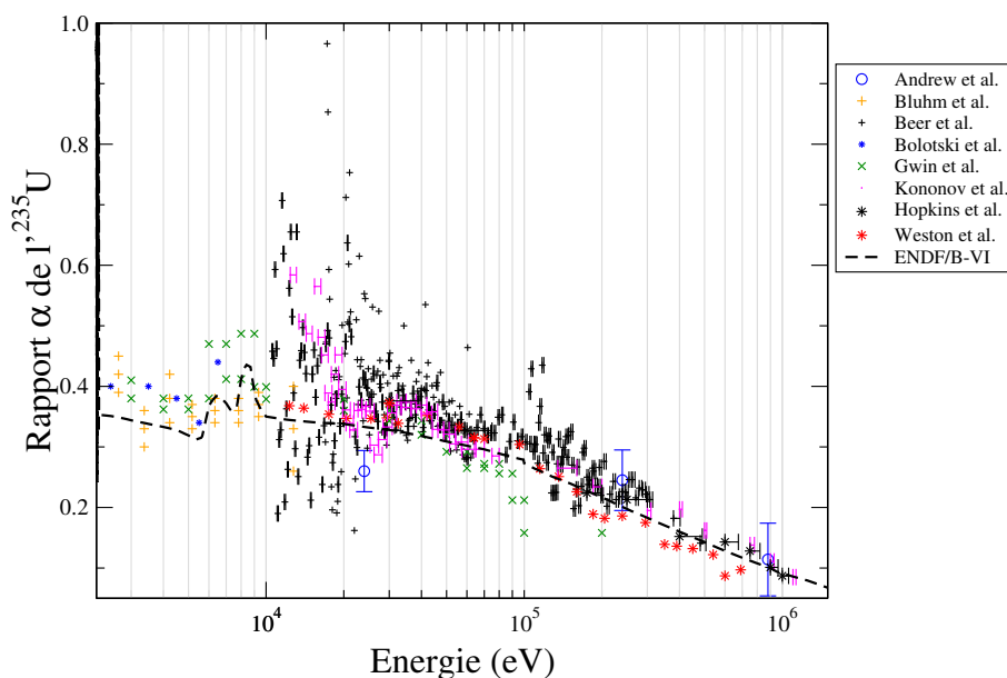
FIG. B.5 – Valeurs expérimentales différentielles du rapport \alpha de l' ^{235}\text{U} répertoriées dans la base EXFOR, comparées à l'évaluation ENDF/B-VI, pour les hautes énergies ( > 2.2 \text{ keV} ), suite.
