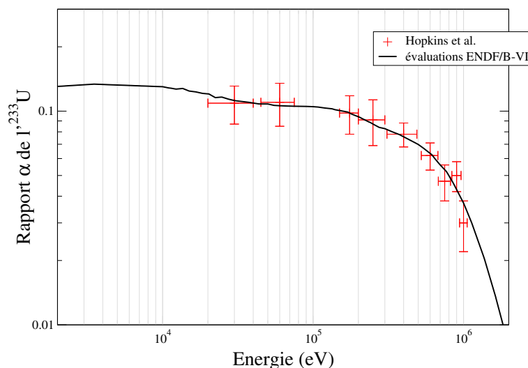
FIG. B.11 – Valeurs expérimentales différentielles du rapport \alpha de ^{233}\text{U} répertoriées dans la base EXFOR, comparées à l'évaluation ENDF/B-VI pour des énergies supérieures à 2 keV.
