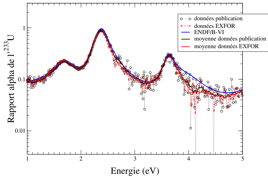
FIG. B.16 – Rapport \alpha de 1^{233}\text{U} entre 1 eV et 5 eV.
