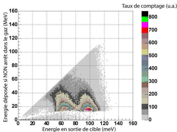
FIG. D.6 – Spectre bidimensionnel “Energie en sortie de cible - Energie déposée Si NON Arrêt dans le gaz” pour le cas de la chambre à fission carrée finale. P_{\text{gaz}} = 0.5 bar.
