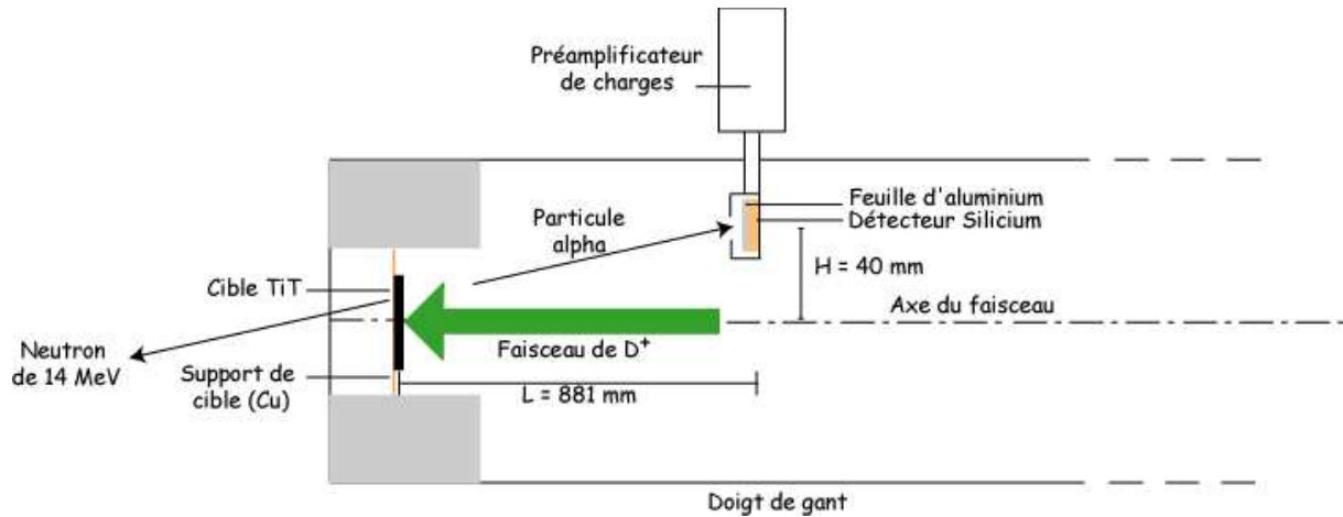
FIG. 3.9 – Schéma simplifié (échelle non respectée) du monitoring grâce au détecteur semi-conducteur Silicium.
