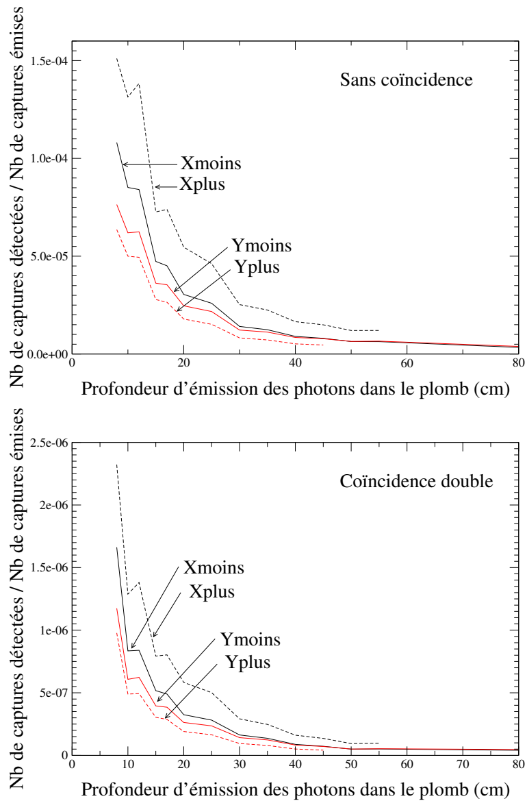
FIG. 9.8 – Nombre d'événements de capture attendus dans les détecteurs, dans les scintillateurs YAP de 2 mm d'épaisseur, par rapport au nombre d'événements de capture émis. Le résultat est représenté sans coïncidence imposée dans la figure du haut et en coïncidence double, dans la figure du bas. Ce taux est représenté selon les 2 directions X et Y prises en compte et en fonction de la profondeur de plomb prise en compte. Les axes X et Y sont représentés sur la figure 9.7.
