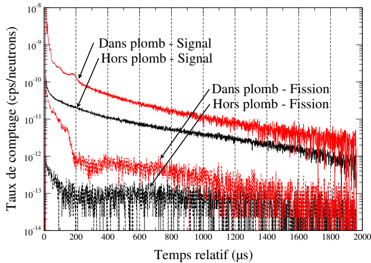
FIG. 9.4 – Spectres en temps relatif des 8 scintillateurs YAP de 2 mm d'épaisseur en coïncidence double pour le signal (mesure avec les cibles d' 235 U) et la fission, lorsque le dispositif expérimental est dans le bloc de plomb ou à l'extérieur.
