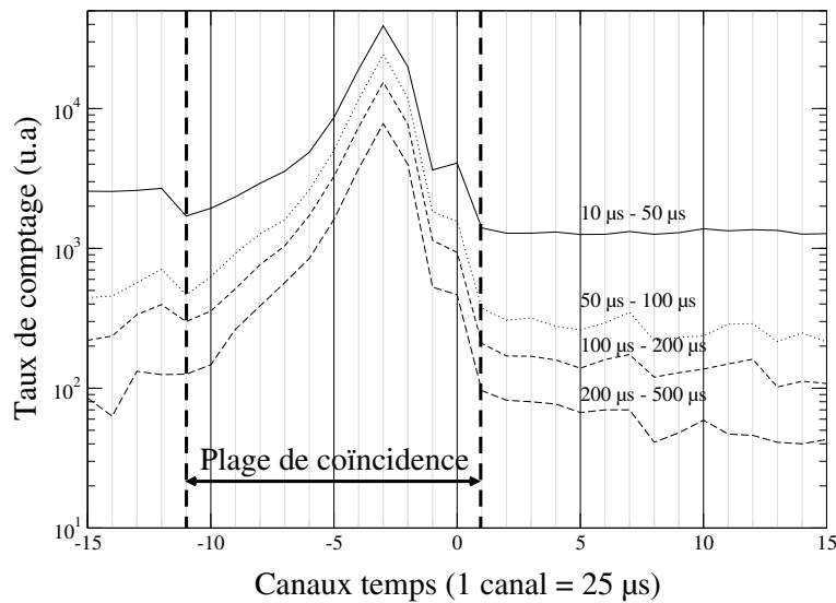
FIG. 7.6 – Distributions de la différence entre le temps d'un événement en single dans les scintillateurs YAP et le temps d'un événement de fission, pour différentes plages en temps relatifs. La plage de coïncidence choisie en conséquence est représentée sur le graphique.
