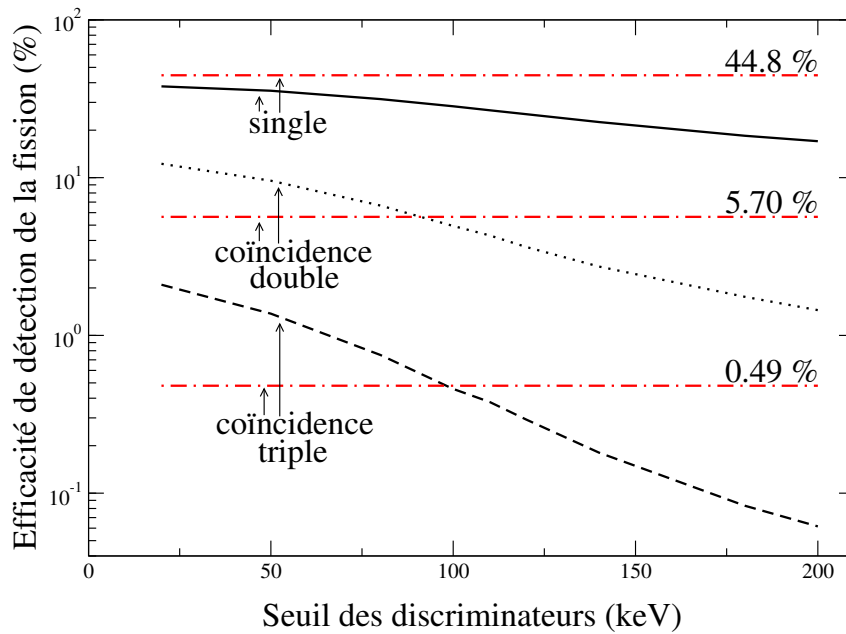
FIG. 8.6 – Efficacité de détection de la fission calculée avec GEANT4 en fonction du seuil des discriminateurs et de la coïncidence imposée. Les courbes constantes dont la valeur est spécifiée sur les graphiques correspond aux valeurs expérimentales. Les efficacités sont représentées pour le cas “10 mm” (en haut) et “2 mm” (en bas).
