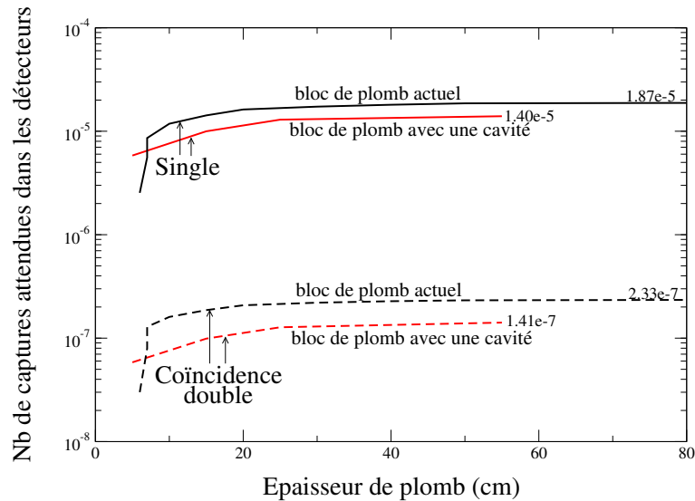
FIG. 10.4 – Nombre d'événements de capture détectés dans les scintillateurs YAP de 2 mm d'épaisseur sans coïncidence (courbe pleine) et en coïncidence double (courbe pointillée), par rapport au nombre d'événements de capture total émis dans le bloc de plomb. Les calculs ont été effectués avec le bloc de plomb présentant une cavité de 25 cm de côté autour des détecteurs et avec le bloc de bloc actuel (sans cavité).
