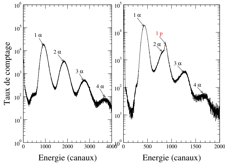
FIG. 3.11 – Exemple de spectres en énergie du détecteur Silicium dans le cas initial avec une source de TiT neuve (à gauche), et dans le cas où, après plusieurs acquisitions, du deutérium s’est implémenté dans la cible de TiT (à droite).
