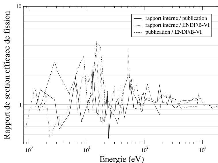
FIG. B.12 – Rapport des section efficace de fission de ^{233}\text{U} , entre le rapport interne ORNL et la publication, entre le rapport interne ORNL et l'évaluation ENDF/B-VI, et entre la publication et l'évaluation ENDF/B-VI.
