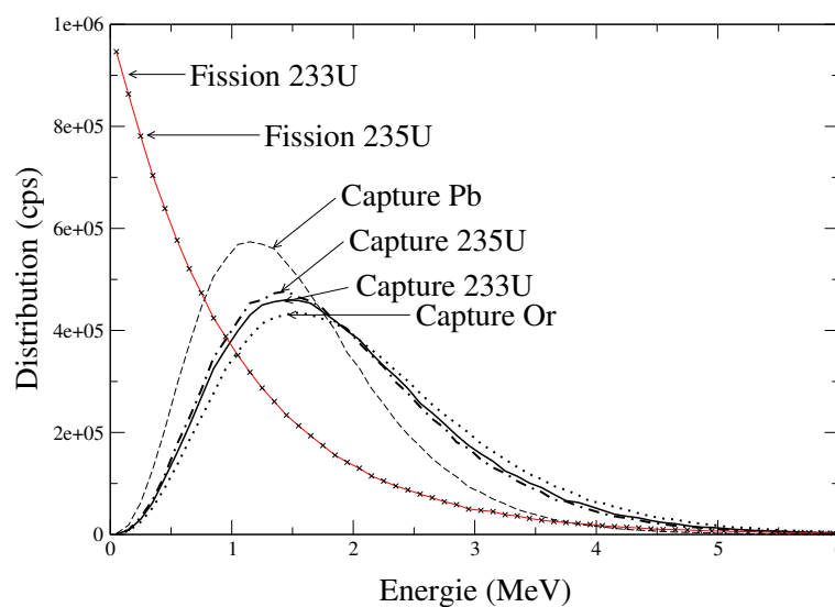
FIG. 6.8 – Distribution en énergie des photons gamma émis suite à une capture ou une fission neutronique en fonction de l'élément considéré.
