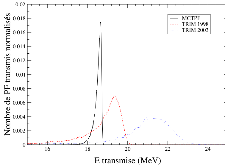
FIG. 5.15 – Spectres d'énergie de sortie de cible de l'élément 145 Ba d'énergie initiale 100 MeV obtenus par TRIM 1998, TRIM 2003 et MCTPF utilisant les tables de parcours données par SRIM 2003. L'épaisseur de la cible est 5 \mu\text{m} .
