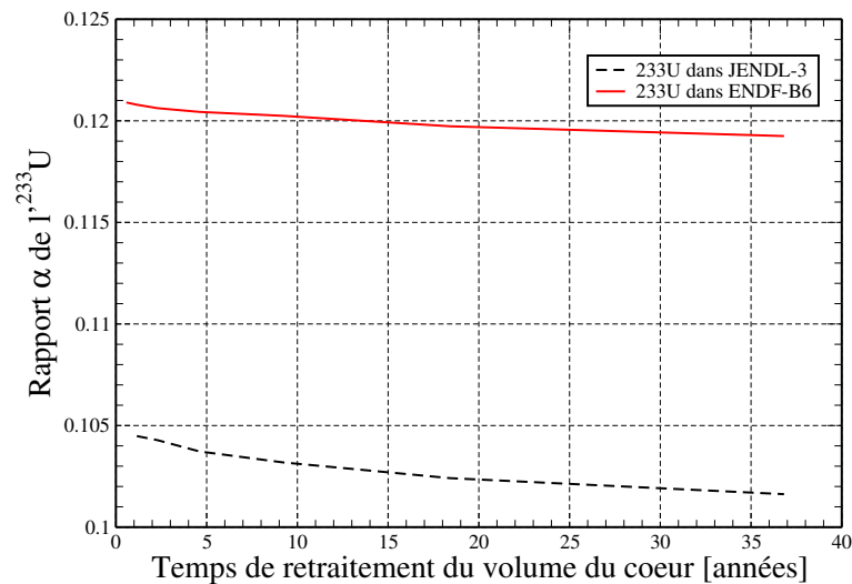
FIG. 2.13 – Comparaison du rapport \alpha de l' ^{233}\text{U} en fonction du temps de retraitement du volume du coeur, et en fonction de l'évaluation utilisé pour l' ^{233}\text{U} .
