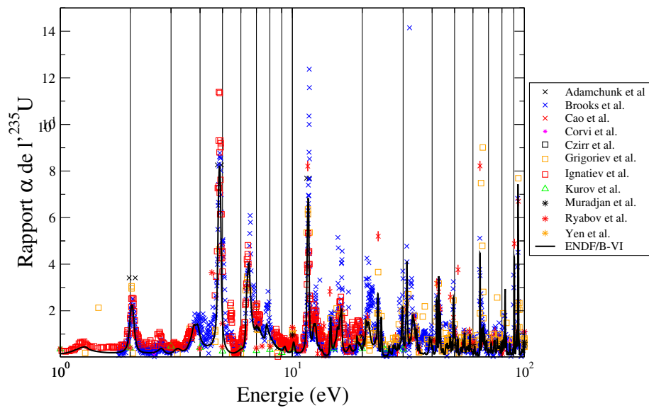
FIG. B.2 – Valeurs expérimentales différentielles du rapport \alpha de ^{235}\text{U} répertoriées dans la base EXFOR, comparées à l'évaluation ENDF/B-VI, pour des énergies comprises entre 1 eV et 100 eV.
