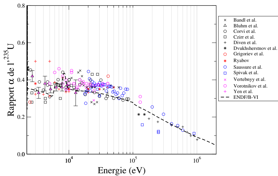
FIG. B.4 – Valeurs expérimentales différentielles du rapport \alpha de 1^{235}\text{U} répertoriées dans la base EXFOR, comparées à l'évaluation ENDF/B-VI, pour les hautes énergies (> 2.2 keV). Au vu de la quantité de données et afin de rendre plus lisible les courbes, les valeurs expérimentales ont été représentées sur deux graphiques.
