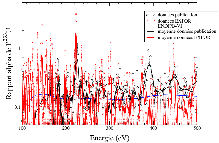
FIG. B.20 – Rapport \alpha de ^{233}\text{U} entre 100 eV et 500 eV.
