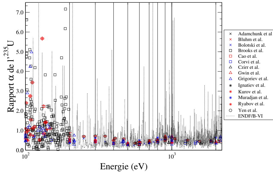
FIG. B.3 – Valeurs expérimentales différentielles du rapport \alpha de 1^{235}\text{U} répertoriées dans la base EXFOR, comparées à l'évaluation ENDF/B-VI, pour des énergies comprises entre 100 eV et 2.2 keV.
