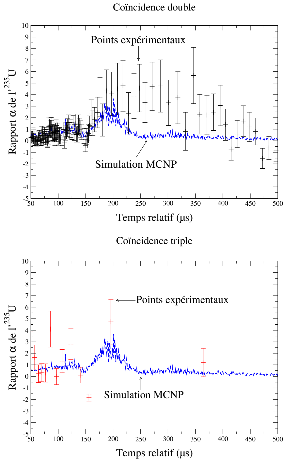
FIG. 8.18 – Comparaison du rapport \alpha de 1^{235}\text{U} obtenu expérimentalement avec celui obtenu par simulation MCNP, pour une coïncidence double (en haut) et triple (en bas). Les simulation MCNP, prenant en compte la composition exacte des cibles, utilisent les évaluations ENDF/B-VI.
