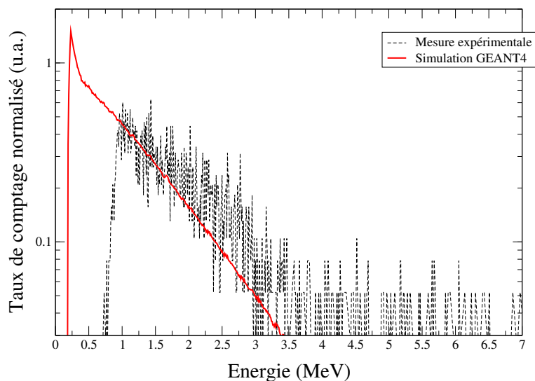
FIG. 10.2 – Comparaison entre le spectre "énergie" expérimental et celui obtenu avec GEANT4 dans le cas d'une cible d'or.
