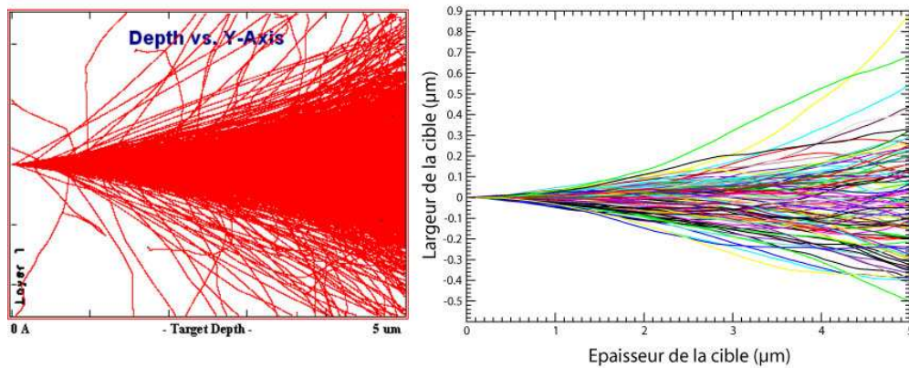
FIG. 5.17 – Trajectoires dans la cible du produit de fission ^{145}\text{Ba} (épaisseur de cible : 5 \mu\text{m} , énergie initiale : 100 MeV) obtenues par TRIM à gauche et par MCTPF à droite.
